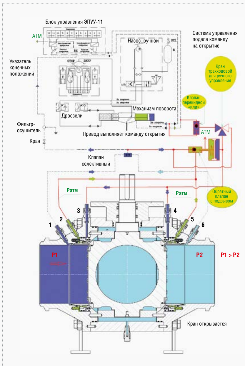
Рис. 12. Схема электропневмогидравлическая «УМНОГО» крана – открытие (закрытие)
