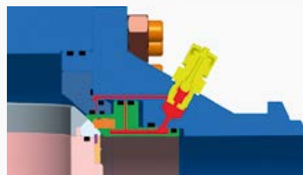
Рис. 16. Подвод уплотнительной смазки в зону уплотнительных колец двухступенчатого поршня
