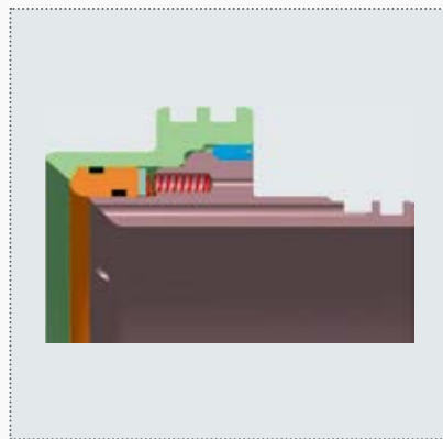
Рис. 8. Конструкция разборного седла с подвижным уплотнительным элементом
