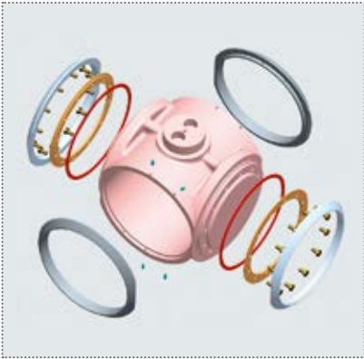
Рис. 10. Кольца могут быть легко демонтированы с запорного органа для замены или ремонта.
