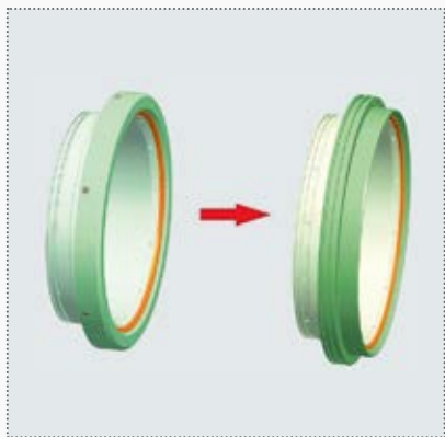
Рис. 6. Замена № 1 – в «УМНЫЙ» кран установлены сёдла в виде кольцевого двухступенчатого поршня.
