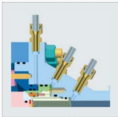
Рис. 7. Расположение каналов в патрубке «УМНОГО» крана, позволяющее управлять седлом
