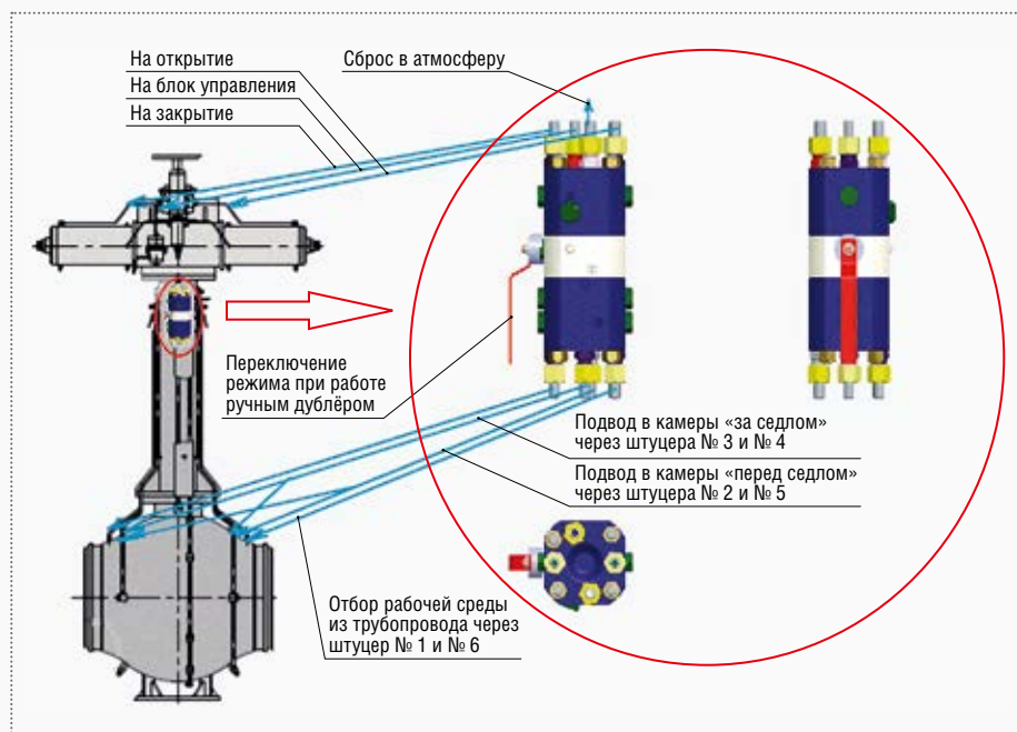
Рис. 17. Пример установки компактного коммутатора на магистральном шаровом кране подземного исполнения
