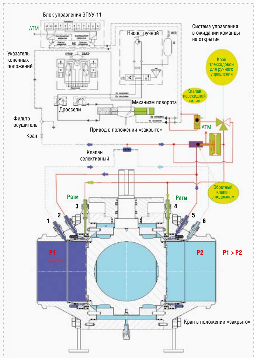
Рис. 11. Схема электропневмогидравлическая «УМНОГО» крана в положении «закрыто». (Черным показаны элементы управления серийным краном, красным – дополнительные элементы обвязки «УМНОГО» крана.)
