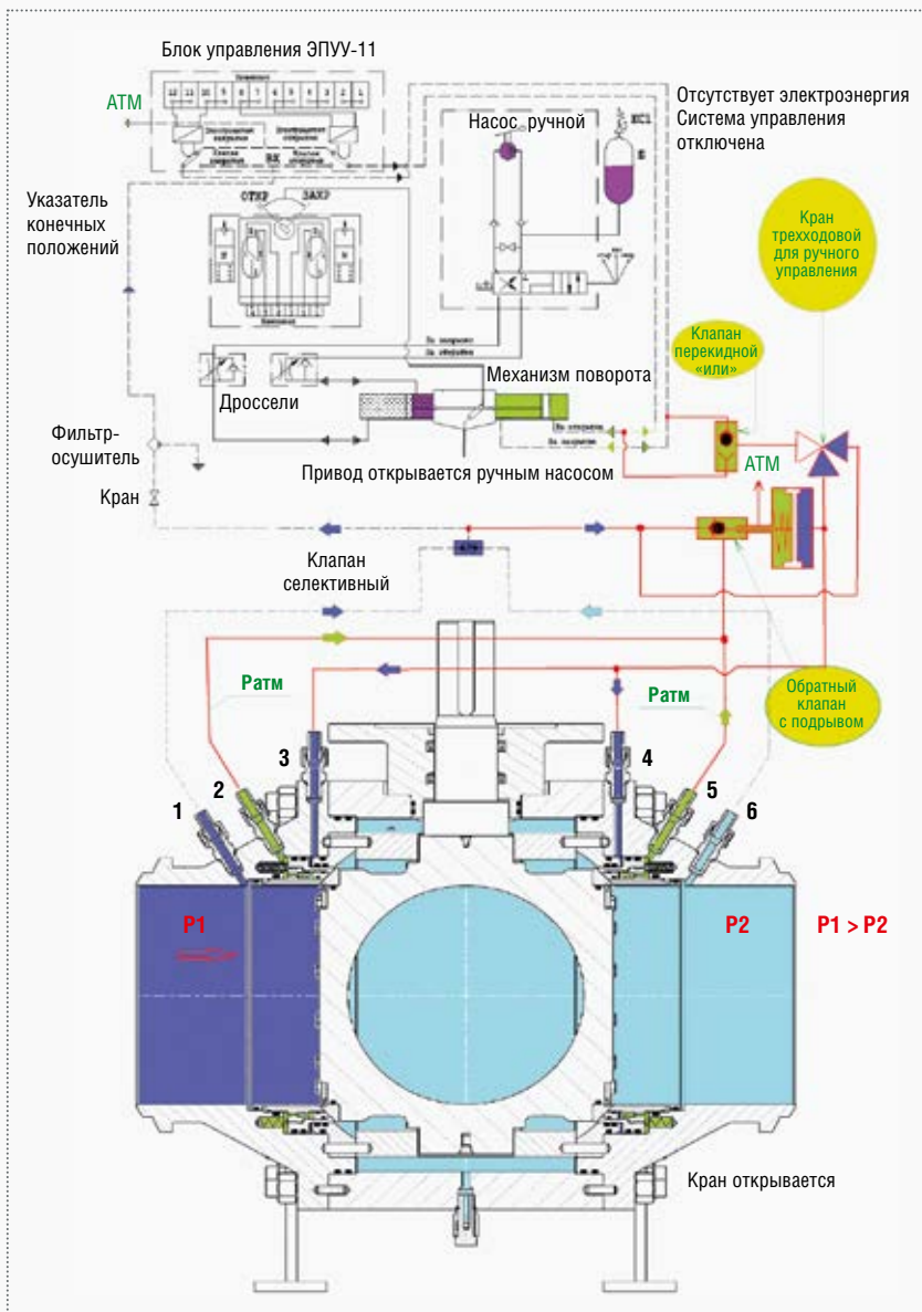
Рис. 14. Схема электропневмогидравлическая «УМНОГО» крана – работа ручным дублиром
