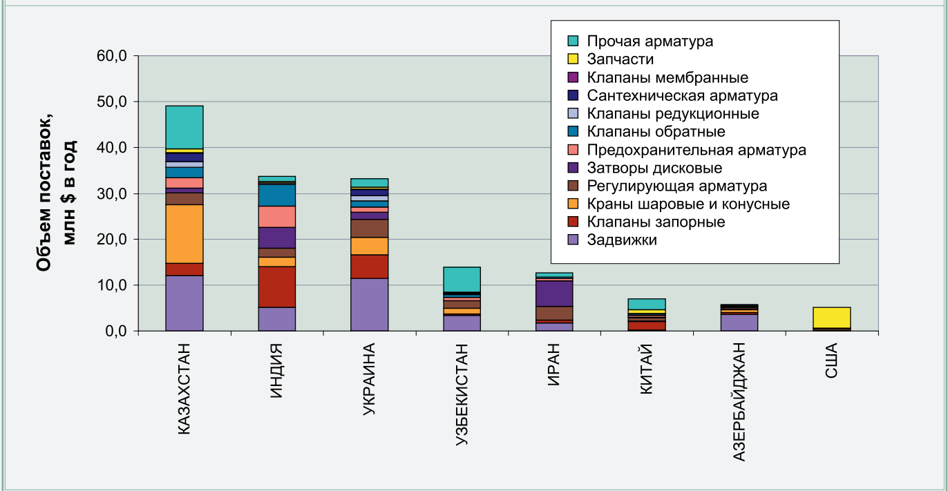
Рис. 14. Ведущие страны-импортеры (объем потребления в 2006 году экспорта из России более 10 млн $). Сегментация по типам
