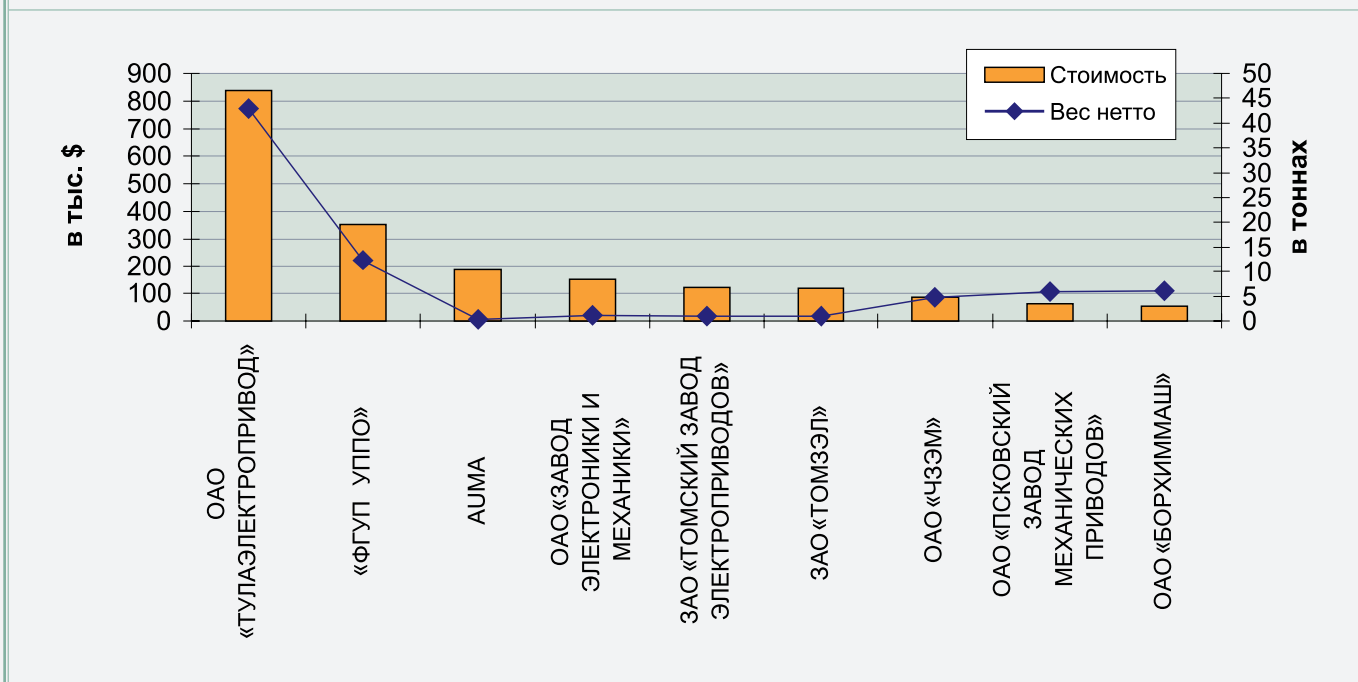
Рис. 22. Сегментация импорта приводов для трубопроводной арматуры в 2006 году по ведущим компаниям-импортерам с объемом импорта более 50 тыс. $ в год
