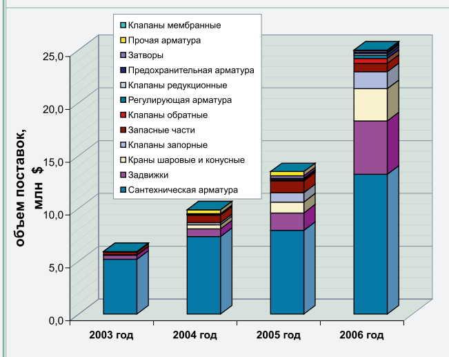
Рис. 17. Китай. Сегментация импорта по типам арматуры за 2003-2006 гг.
