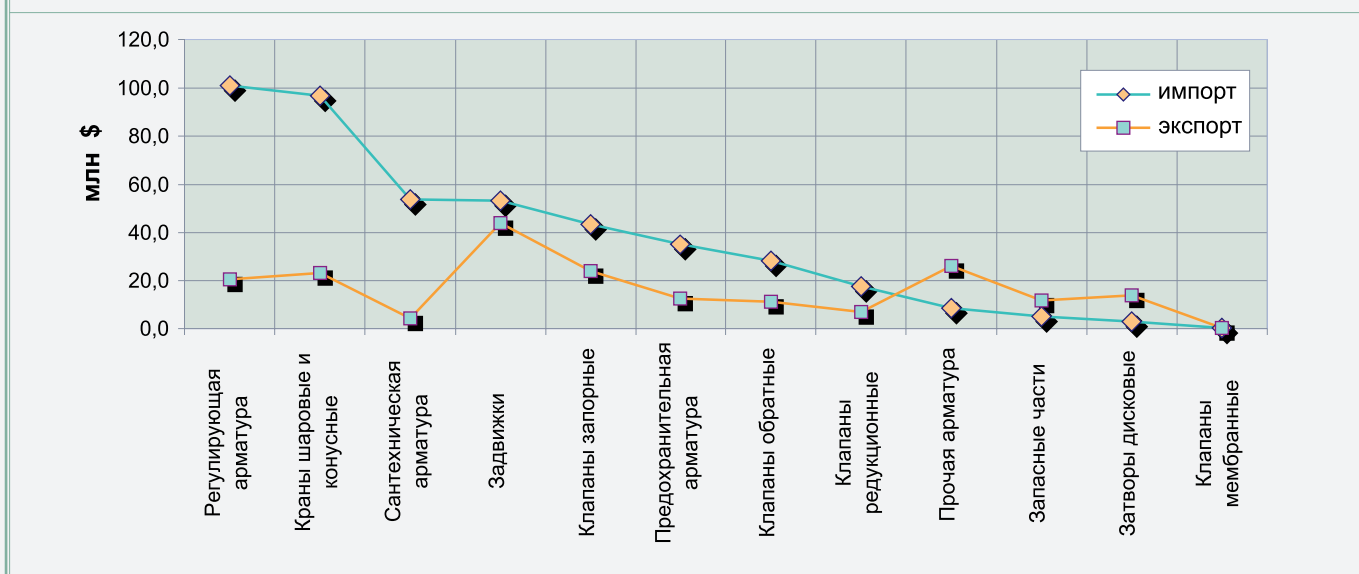
Рис. 16. Соотношение импорта и экспорта в 2006 году. Сегментация по типам арматуры
