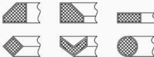
Рис. 1. Типы и внешний вид комбинированных уплотнений
